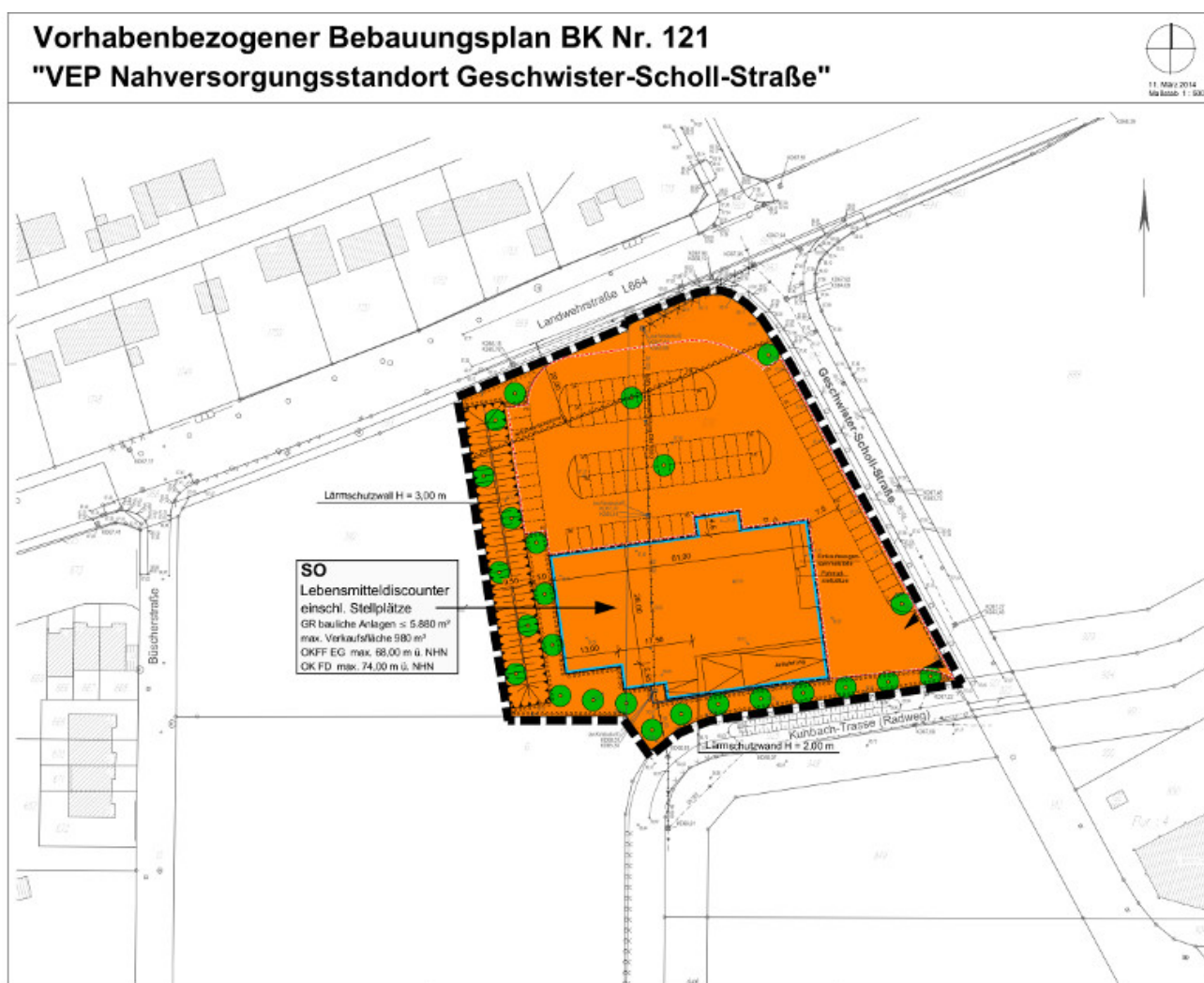
Plan für die Bebauung des Eckgrundstücks
